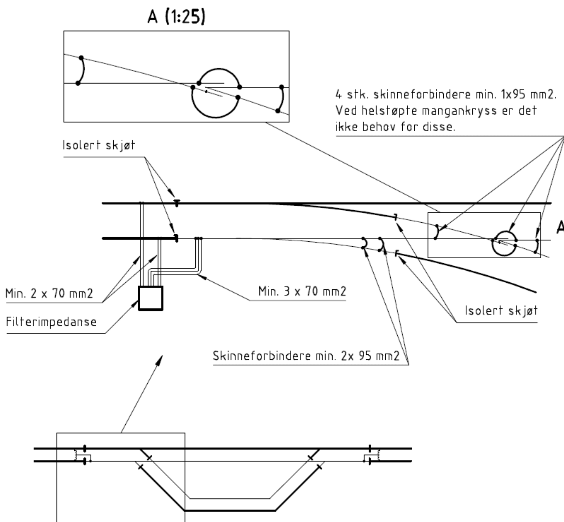
Figur 12.4 Eksempel på bruk av skinneforbindere ved veksler på stasjoner
