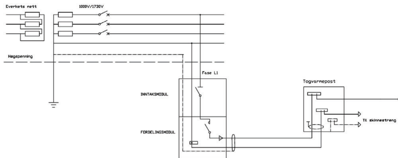
Figur 6.3 Eksempel på prinsipp for 50 Hz togvarmeanlegg med 1000 V /1730 V transformator, 1000 V inntaksmodul, én fordelingsmodul og én togvarmepost.
