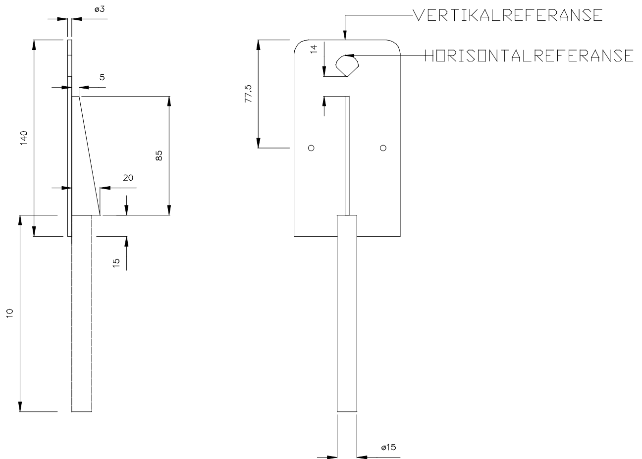
Figur 13.a.1 Horisontalt VUL-merke
