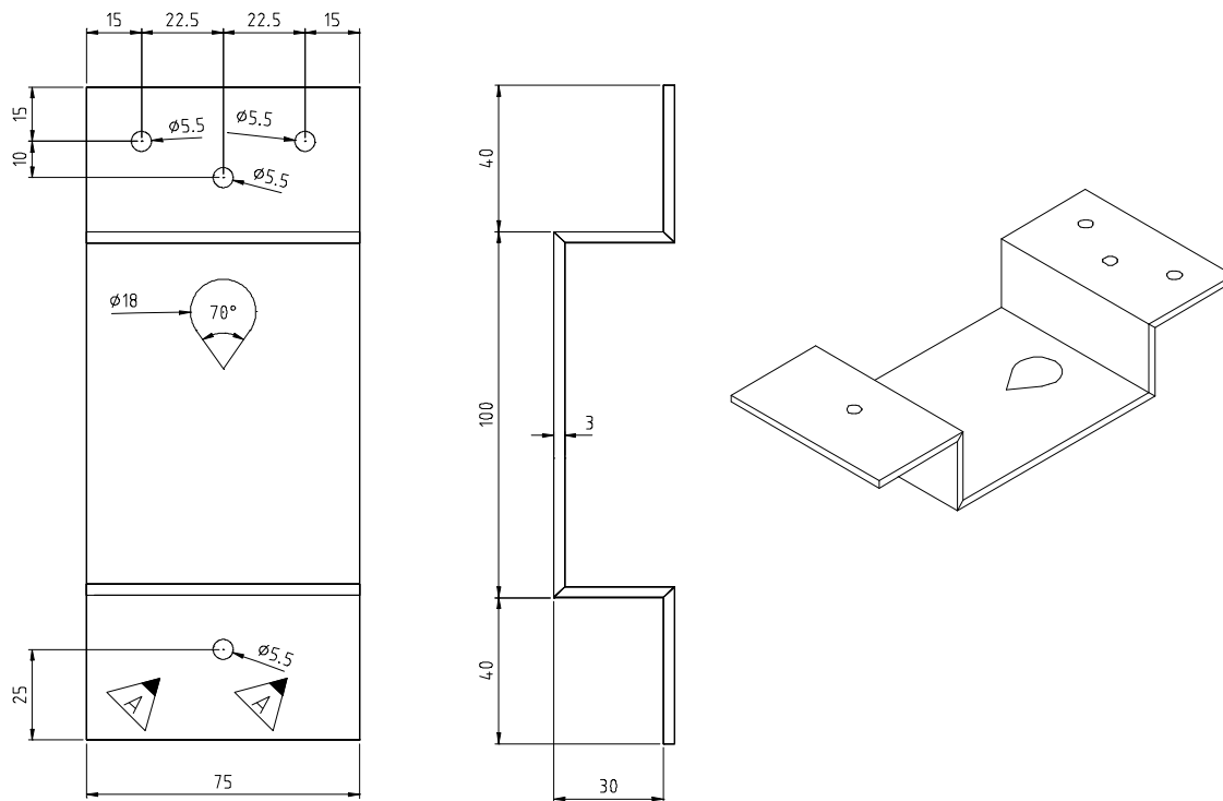
Figur 13.a.2 Vertikalt VUL-merke
