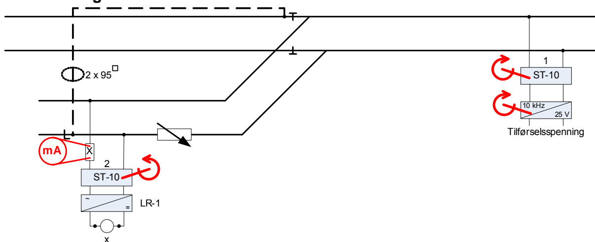
Figur 7.g.1 Justering av 10 kHz sporfelt
