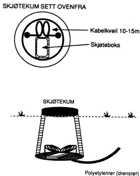
Figur 1, skjøt plassert i skjøtekum.
