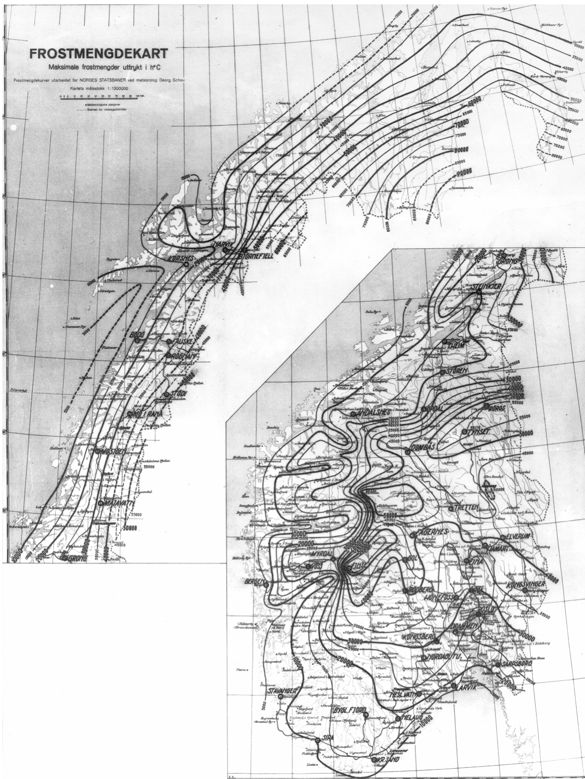
Figur 9.2 Maksimale frostmengder for Norge
