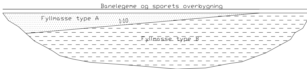
Figur 6.3 Utkiling av masser i fylling. Prinsippskisse av lengdeprofil.
