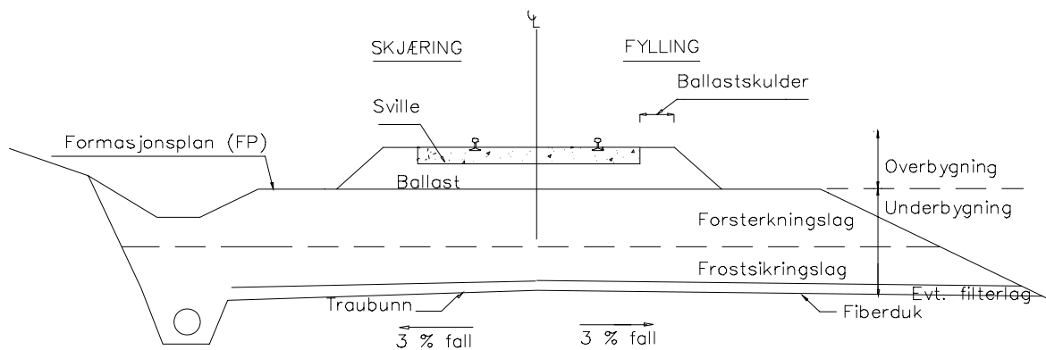
Figur 6.1 Prinsippskisse for oppbygging av jernbanefylling og -skjæring
