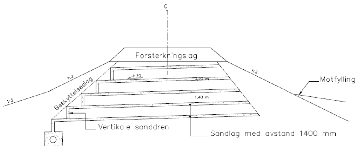
Figur 6.4 Prinsippskisse av leirfylling
