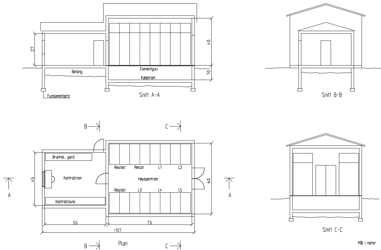
Figur 6.1 Typisk plan og snitt av koblingshus
