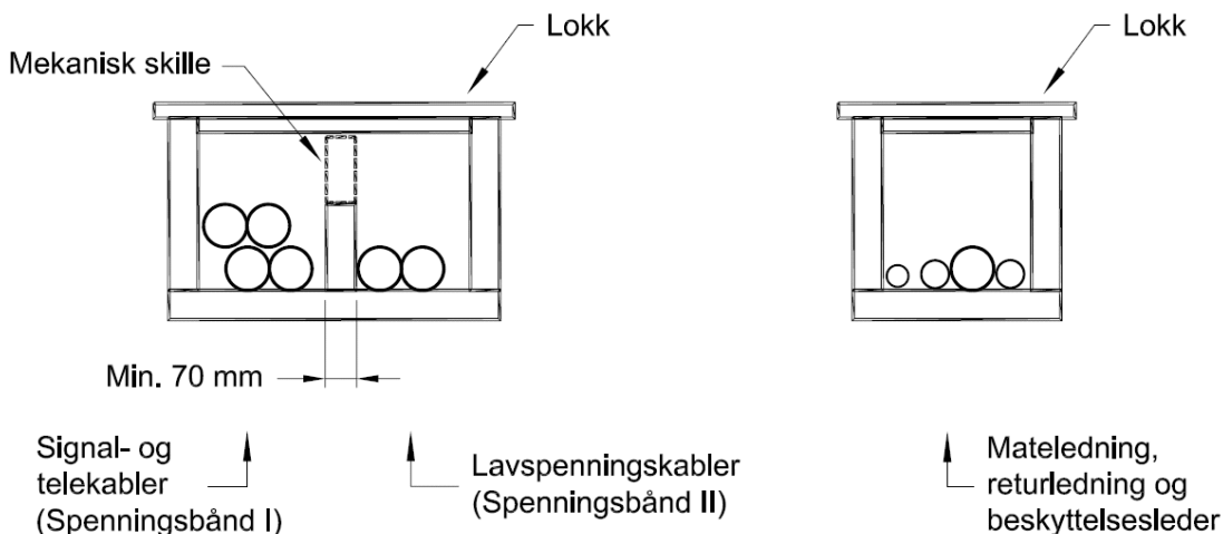
Figur 5.3 Eksempel 1. Tillatt konfigurasjon av kabler i kabelkanal som oppfyller kravene i tabell 5.2.
