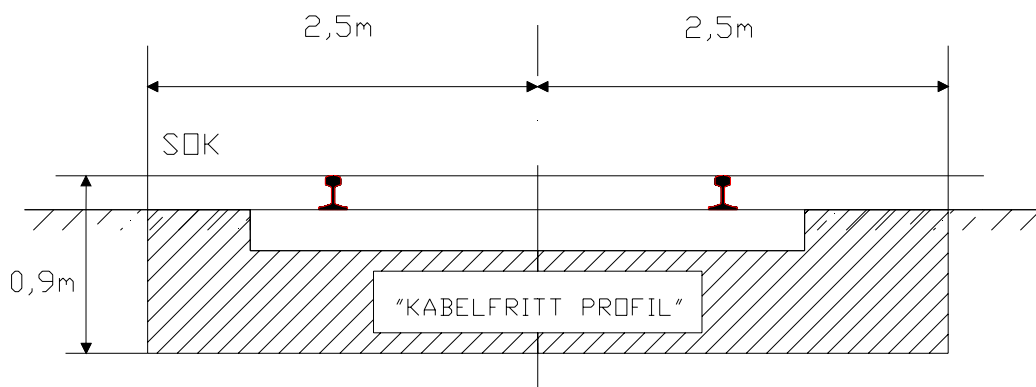
Figur 5.1 Kabelfritt profil.
