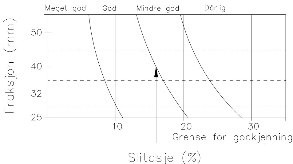
Figur 10.7 Kurvediagram basert på Los Angeles - slitasjetest
