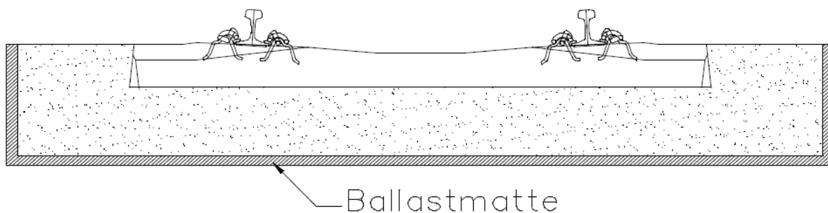
Figur 10.10 Ballastmatte i formasjonsplanet
