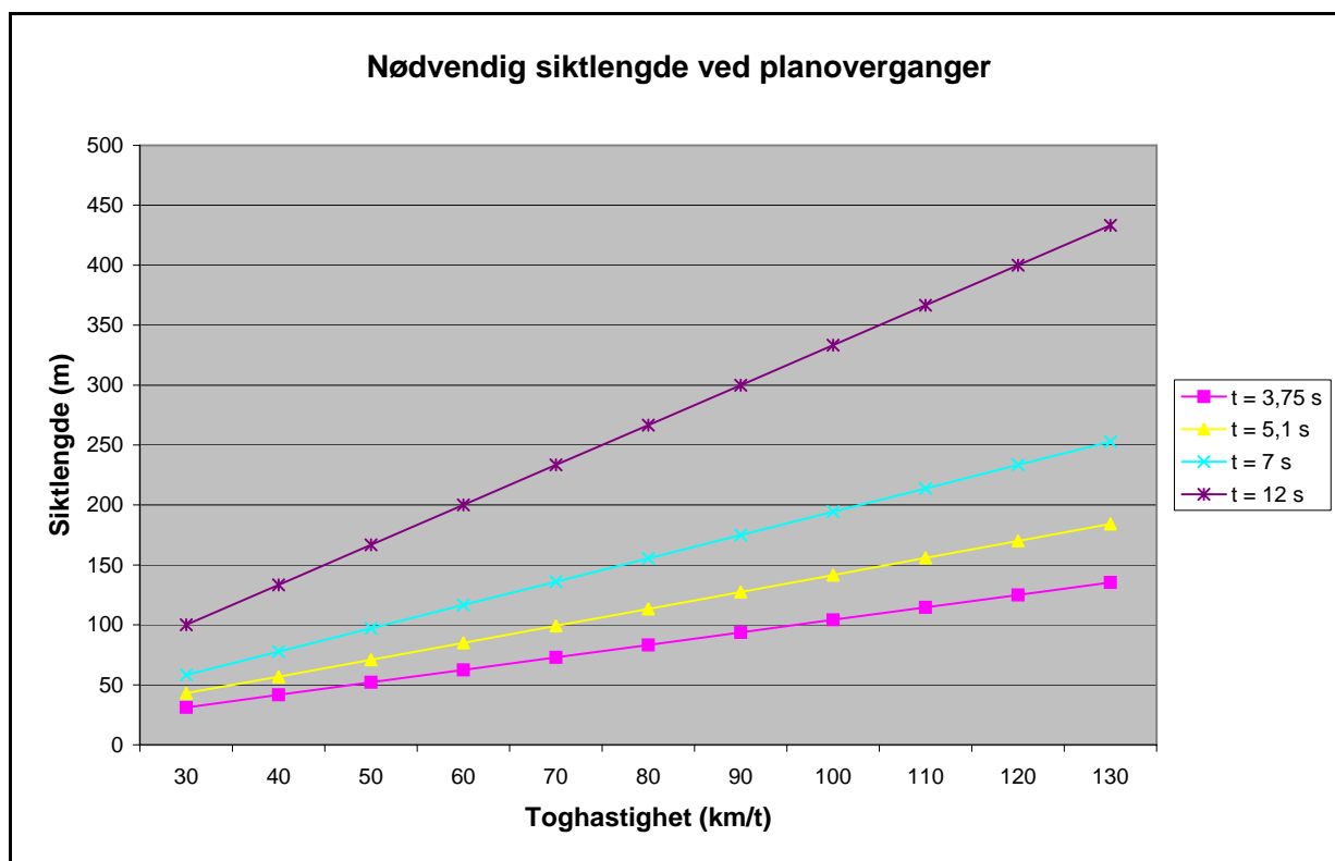
Figur 2 Nødvendig siktlengde ved planovergang
