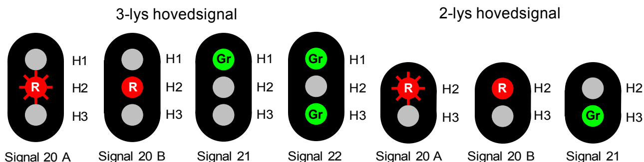
Figur 6.16 Hovedsignal 3-lys - signalbilder
