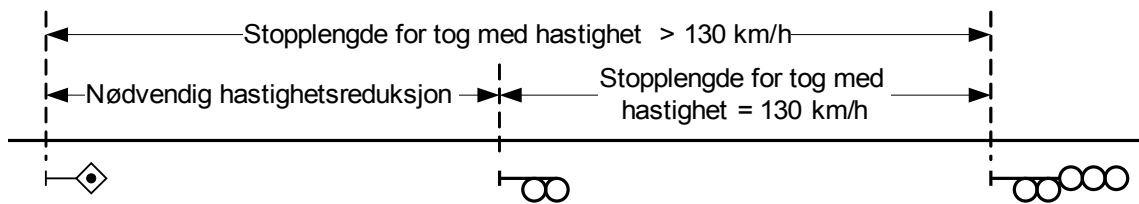
Figur 6.6 Plassering av frittstående forsignal og framskutt forsignal på strekning med kjørehastighet > 130 km/h
