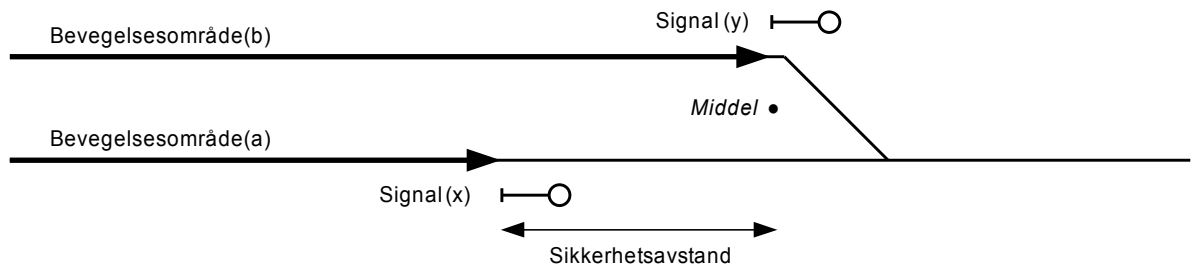
Figur 6.12 Parallele bevegelsesområder
