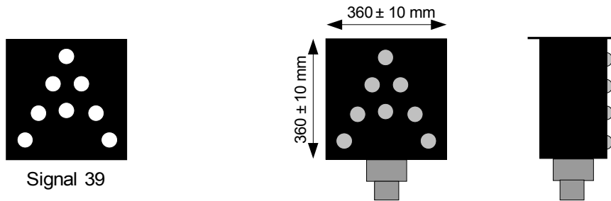
Kjøretillatelse "A-signal" - signalbilde og eksempel på lyssignal
