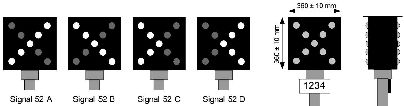
Figur 6.33 Sporvekselsignal for kryssveksel - signalbilder og eksempel på lyssignal
