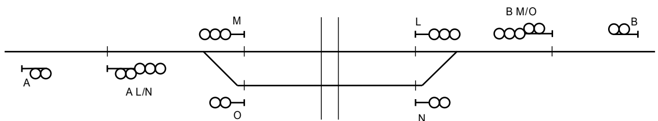
Figur 9.8 Planovergang mellom inn- og utkjørhovedsignalene.
