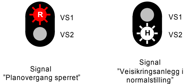
Figur 9.11 Veisignal - Signalbilder
