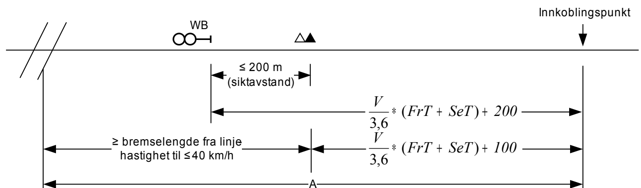
Figur 9.6 Plassering av et innkoblingspunkt på strekning utrustet med FATC
