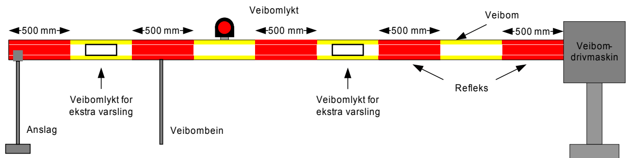
Figur 9.14 Eksempel på veibom
