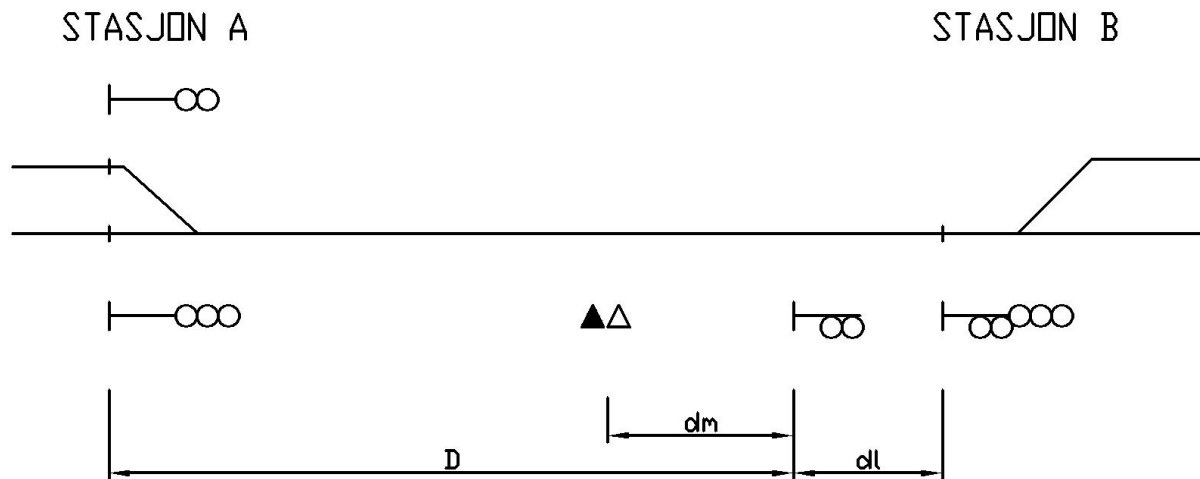
Figur 10.1 Plassering av lenkingsbalisegrupper på linjen
