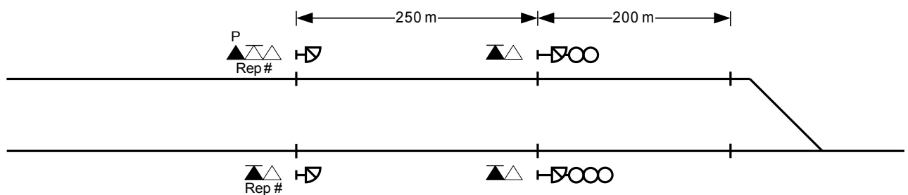
Figur 10.3 Prosjektering av FATC ved samtidige togbevegelser jfr. kap. 6, avsn. 2.2.1, fig. 6.9
