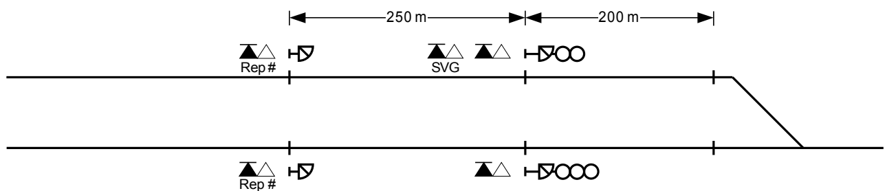
Figur 10.2 Prosjektering av DATC ved samtidige togbevegelser jfr. kap. 6, avsn. 2.2.1, fig. 6.9
