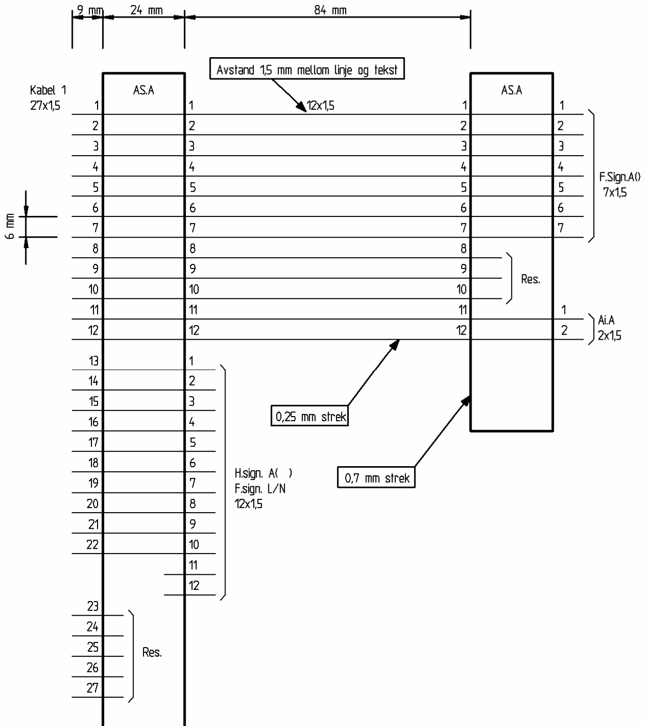
Figur 4.2 Utsnitt av trådfordeling i AS
