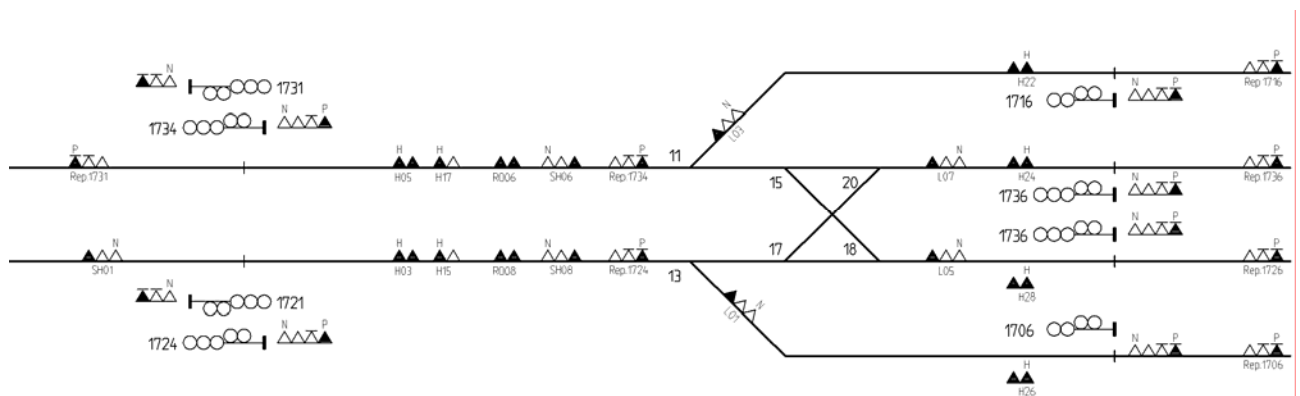
Figur 4.6 Utsnitt av Signal- og baliseplassering for dobbeltspor
