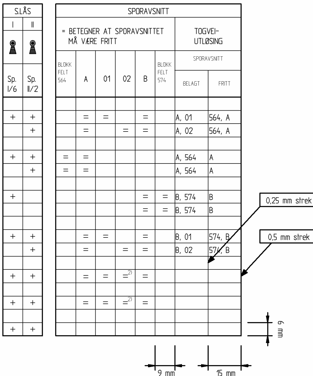
Figur 4.1 Utsnitt av skjematisk plan og forriglingstabell
