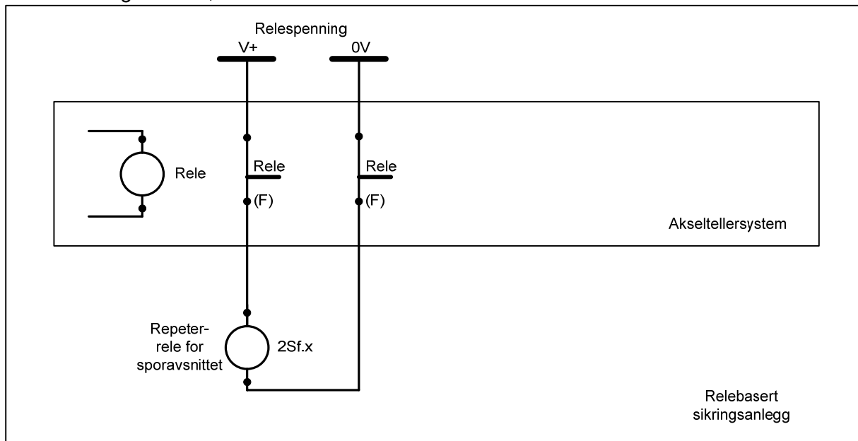
Figur 7.f.15 Grensesnitt mellom akselteller og relebasert sikringsanlegg (m/repeterrele)
