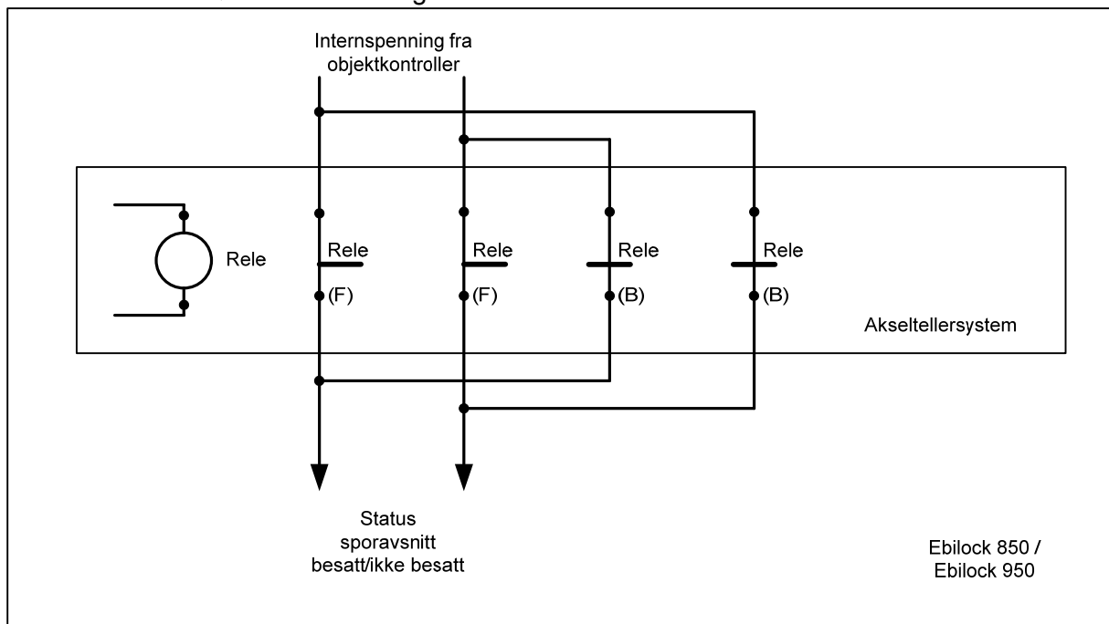
Figur 7.f.19 Grensesnitt mellom akselteller og sikringsanlegg Ebilock 850 og Ebilock 950
