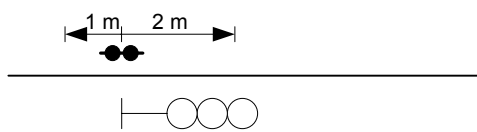
Figur 7.f.8 Hovedsignal eller dvergsignal ved isolert skjøl
