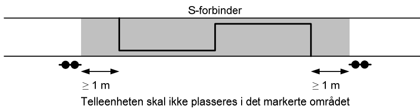
Figur 7.f.6 Avstand fra forbinder (FTG S) til telleenhet
