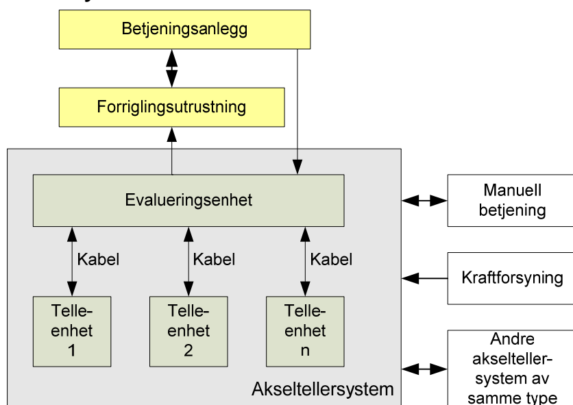
Figur 7.f.1 Systemoversikt akselteller
