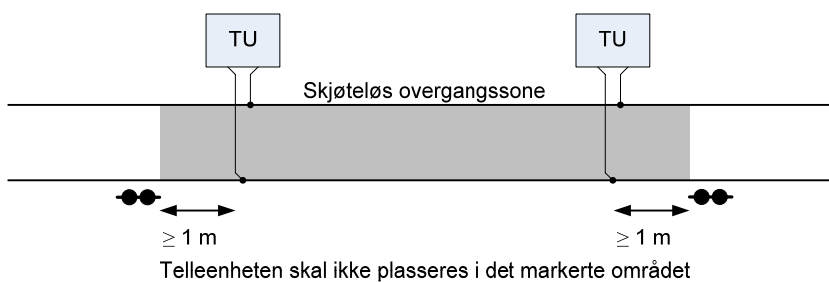
Figur 7.f.7 Avstand fra skjøteløs overgangssone (TI21) til telleenhet
