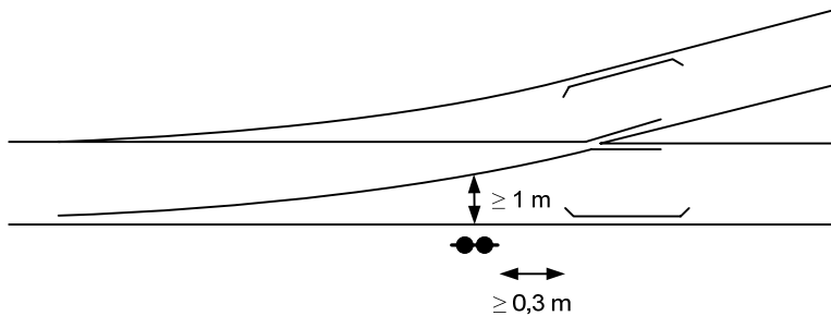
Figur 7.f.5 Avstand fra telleenhet til annen skinne
