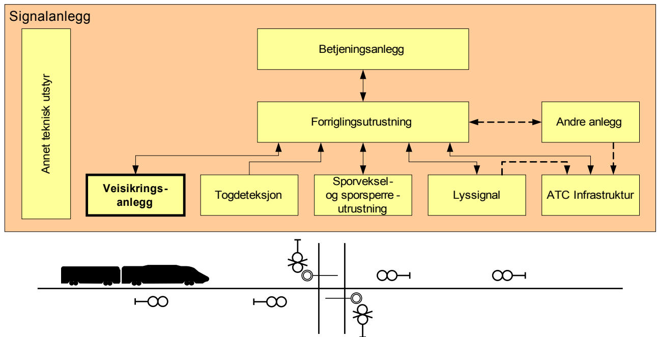
Figur 9.1 Systemoversikt signalanlegg
