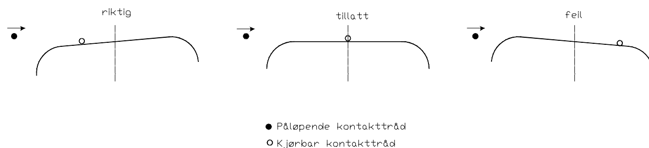
Figur 5.3 Ledningsføring ved sporveksler.
