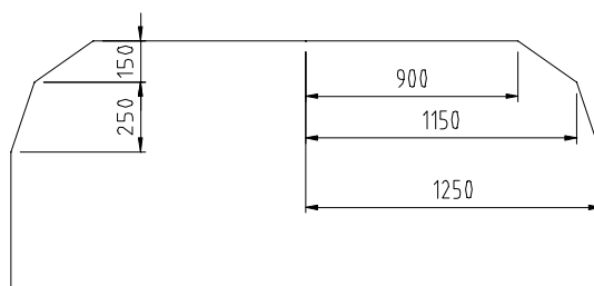
Figur 5.1 Fritt profil for strømavtaker, alle mål i mm.
