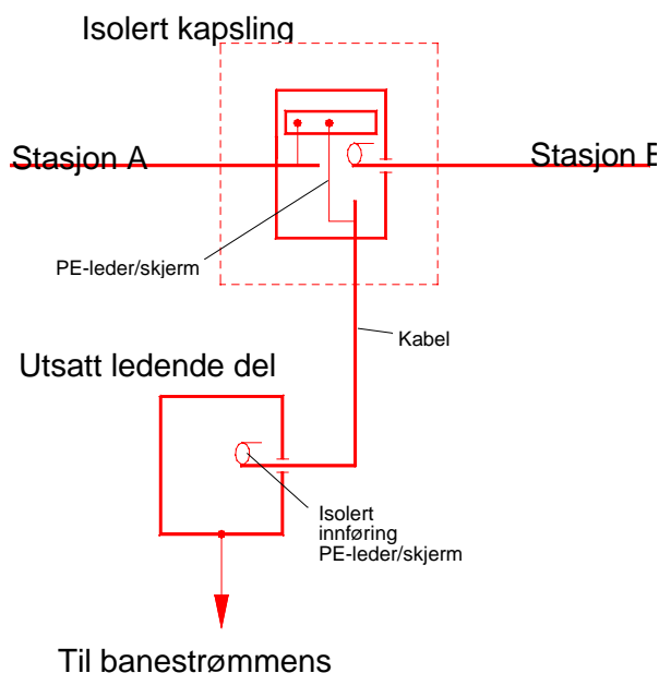
Figur 6.8 Jording, brudd mellom stasjoner
