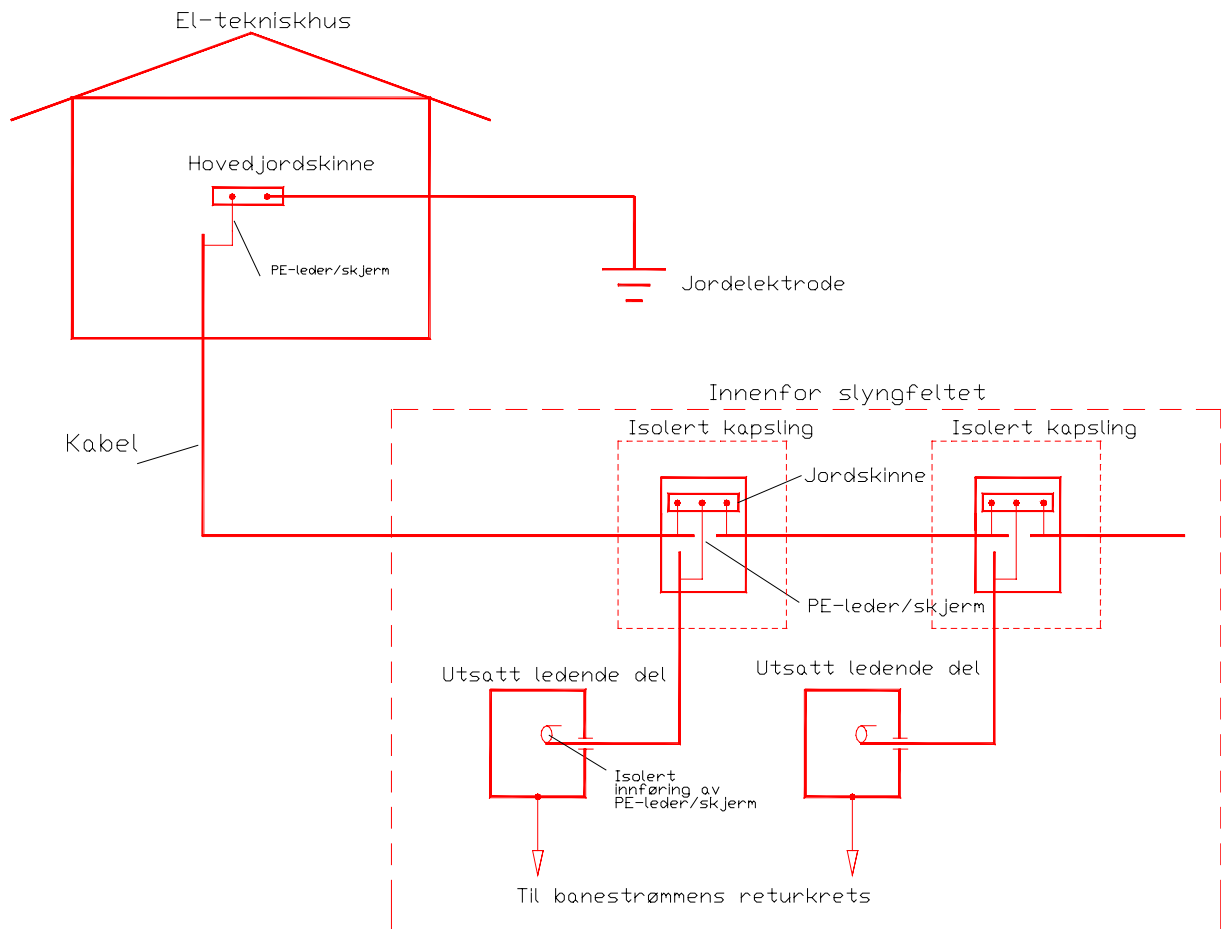
Figur 6.7 Jording av kabler ved innføring i isolerte kapslinger innenfor slyngfeltet Utstyr kan være: signal, drivmaskin, lysmast, etc..
