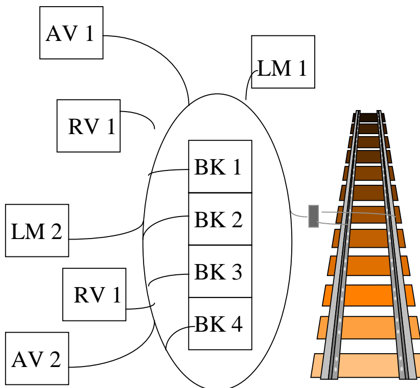
Figur 6.13 Sammenkobling av ledende gjenstander til en større ledende konstruksjon.
