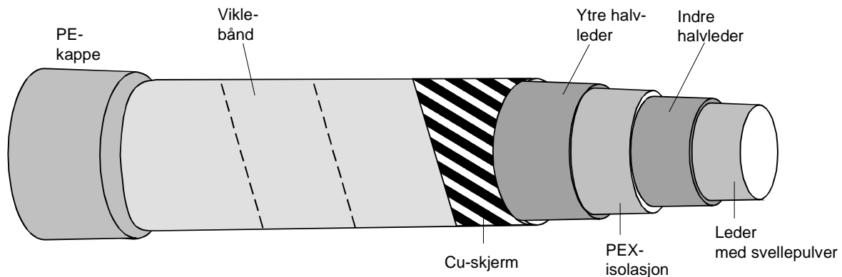
Figur 5.a.2 Langssnitt av 36 kV PEX - kabel
