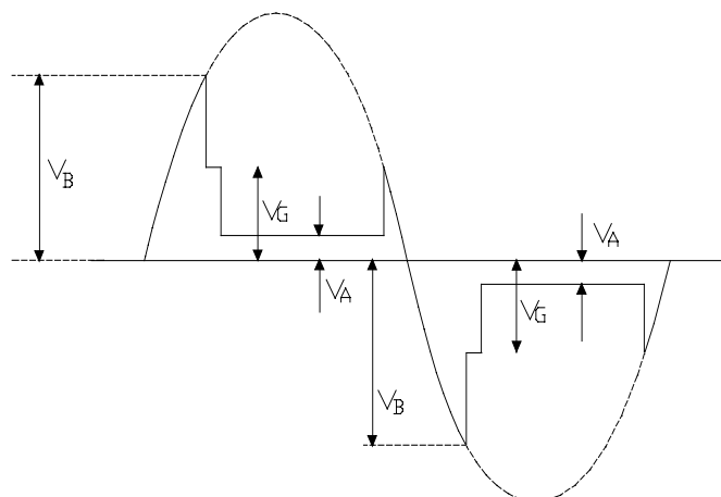
Figur7.a.3 Overspenningsavlederens spenningskarikastikk
