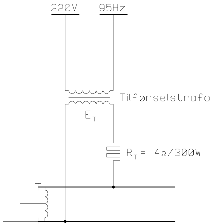
Figur 6.e.7 Tilførselkrets type 3.
