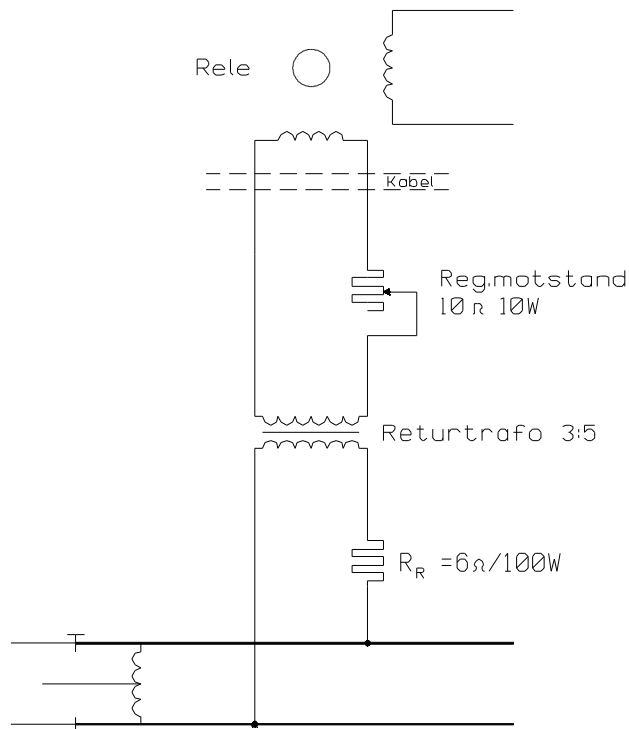
Figur 6.e.11 Returkrets type 4.
