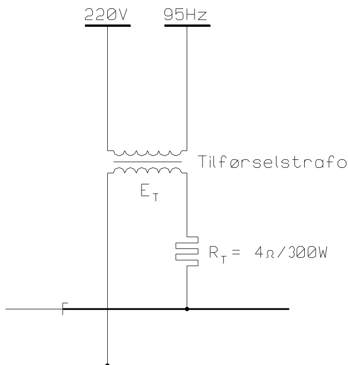
Figur 6.e.4 Tilførselkrets type 2.
