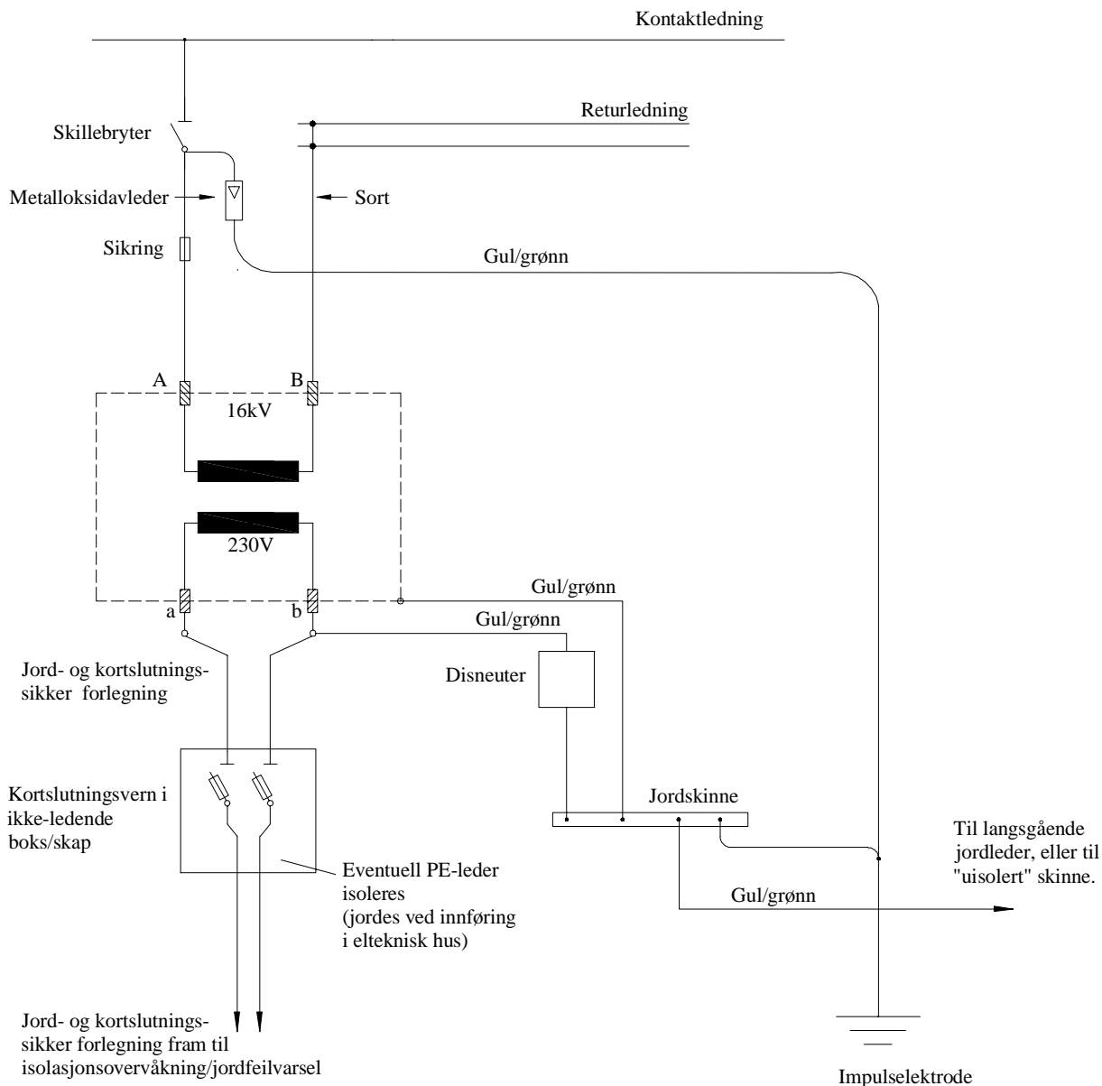
Figur 8.1 Kobling av reservestrømstransformator.
