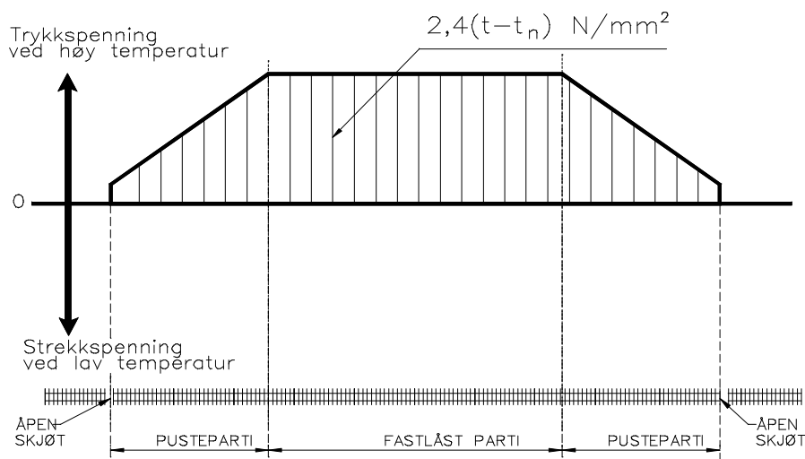
Figur 6.1 Spenninger i helsveist spor
