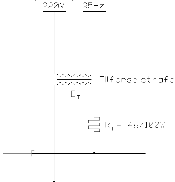
Figur 6.e.1 Tilførselkrets type 1.
