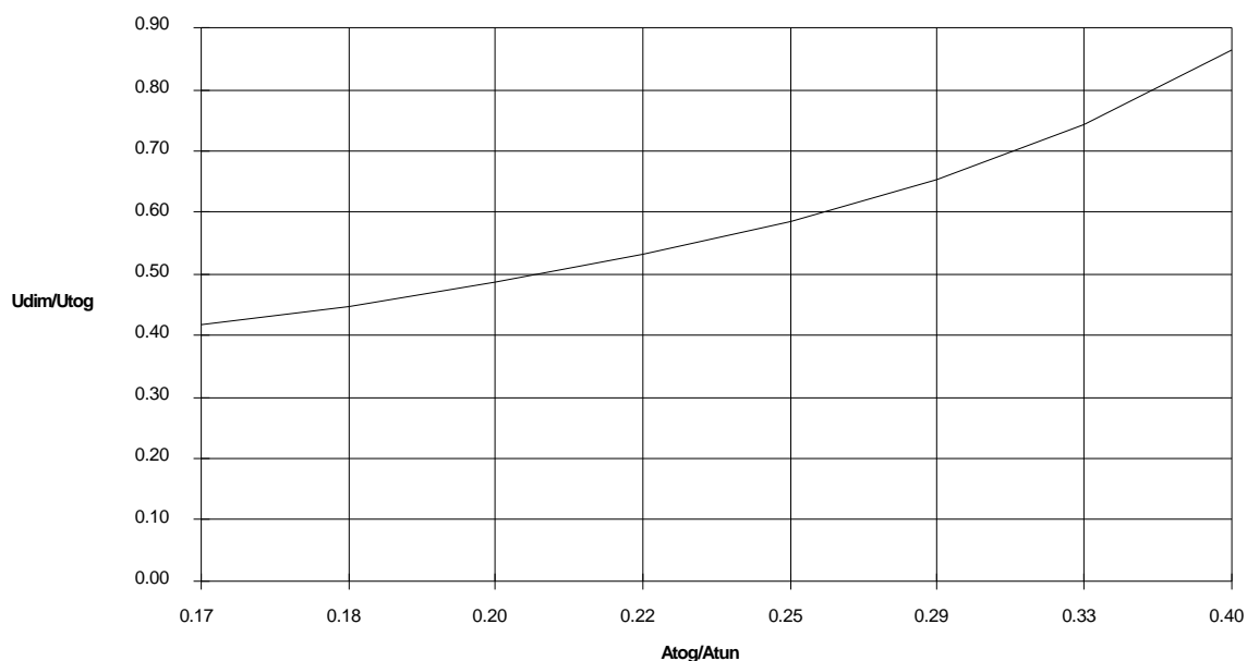
Figur 12.4 Maksimal lufthastighet i enkelt- og dobbeltsporet tunnel
