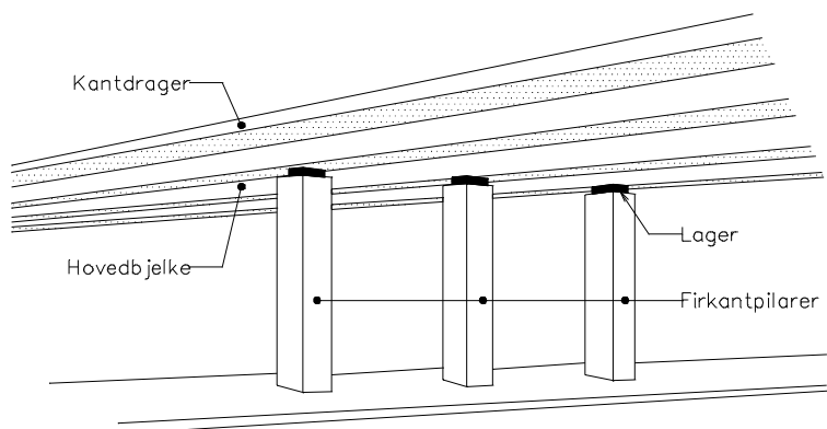
Figur 3.8 Firkantpilarer
