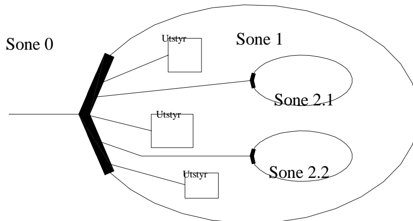
Figur 4.2 Eksempel på jording mellom utstyr i en sone og mellom ulike soner
