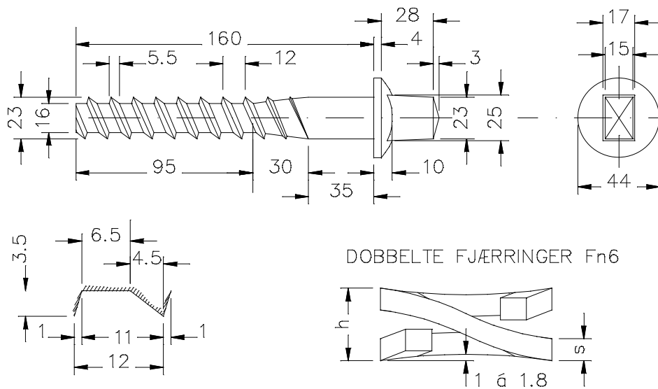
Gjenge-detalj
