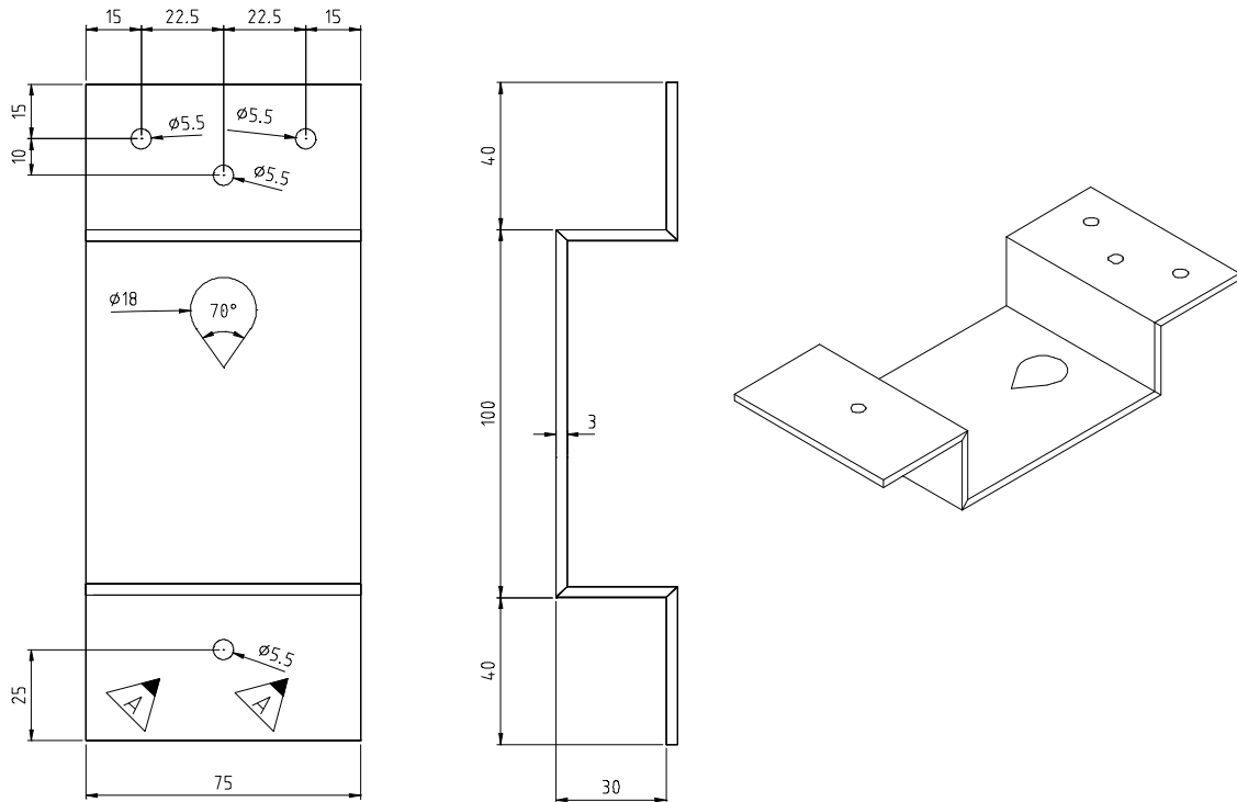
Figur 13.a.2 Vertikalt VUL-merke
