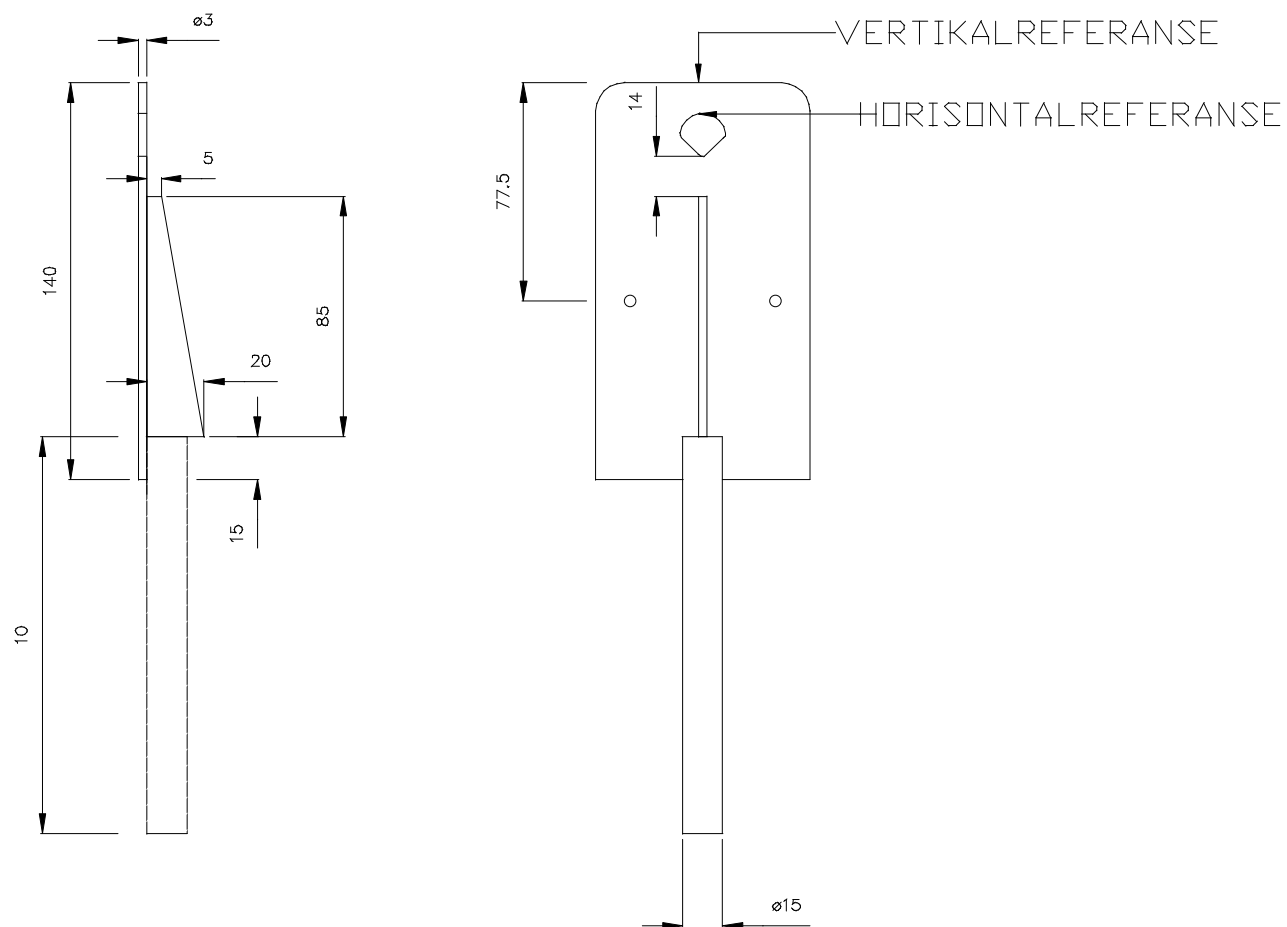
Figur 13.a.1 Horisontalt VUL-merke
