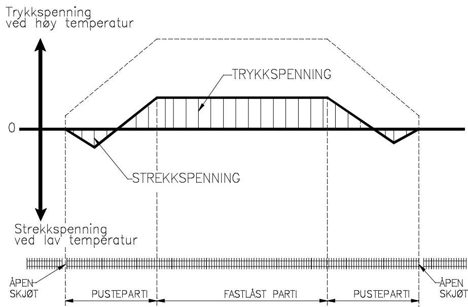
Figur 6.2 Spenninger i pustepartier ved temperaturendringer
