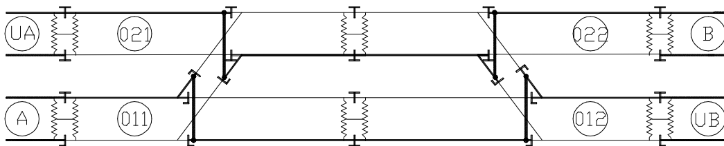
Figur 6.32 Stasjon på dobbeltsporet strekning, elektrifisert bane. Dobbeltisolert m/skinnebruddsdeteksjon. Høyre/venstre hovedspor skal være elektrisk adskilt.
