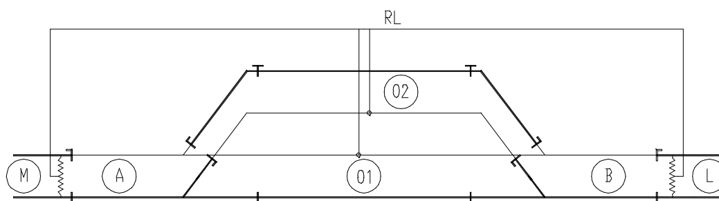
Figur 6.29 2-spors stasjon, elektrifisert strekning. Returleder over stasjon. Enkelt isolert - ikke skinnebruksdeteksjon i spor 1 og 2.
