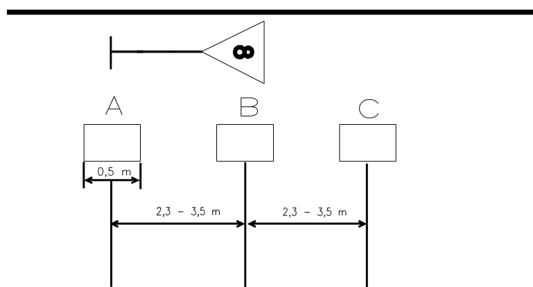
Figur 10.13 Baliseplassering ved hastighetssignaler.
