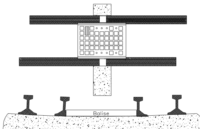
Figur 10.7 Plassering og tilpassing av stor balise i ledeskinner.
