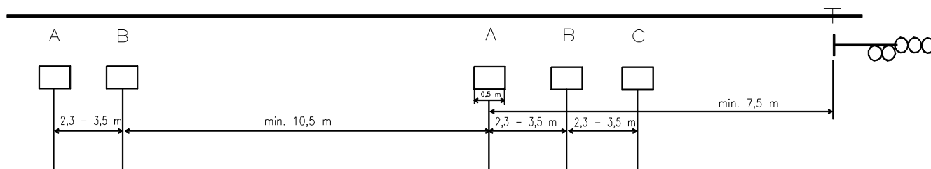
Figur 10.9 Plassering av baliser ved et innkjørhovedsignal.
