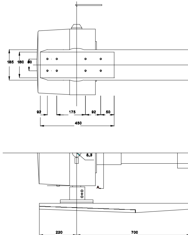
Veibomdrivmaskin type FBD-1 fabrikkat Elektromekano Bredaryd, sett ovenfra og fra siden.
