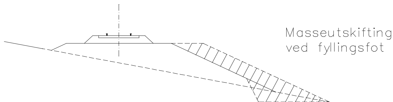
Figur 6.2 Forsterkning av fyllingsfot
