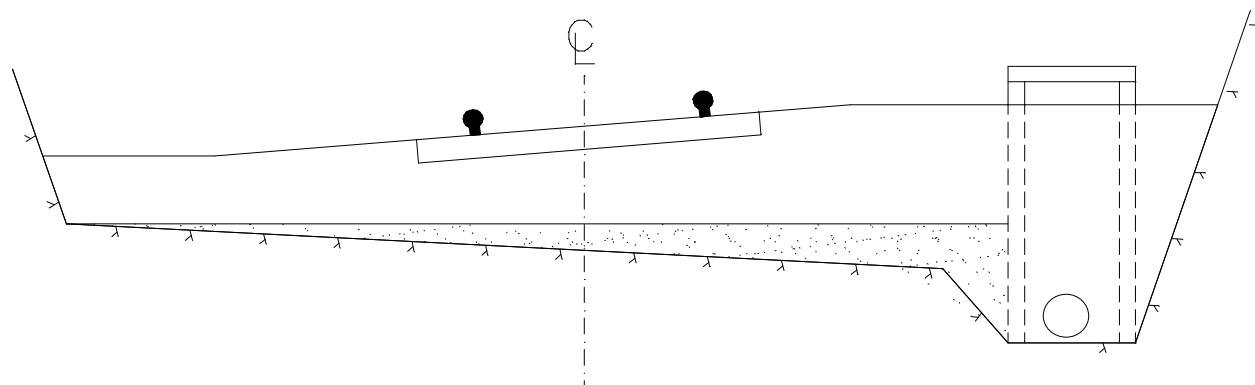
Figur 6.6 Åpen grøft erstattes med rør og kummer
