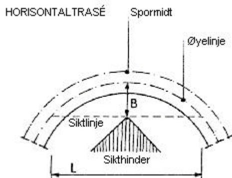
Figur 13.3 Siktforhold i horisontaltrasé
