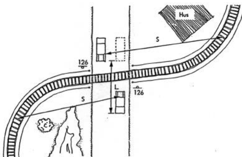
Figur 13.1 Definisjon av siktlengde (S) og den lengde kjøretøyet må kjøre (L)
