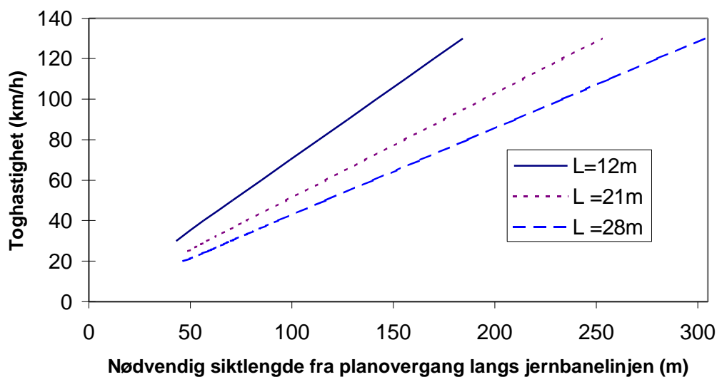
Figur 13.2 Nødvendig siktlengde fra planovergang
