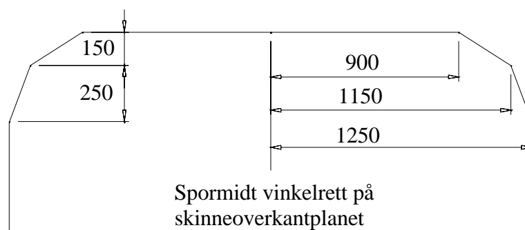
Figur 5.1 Fritt profil for strømavtaker, alle mål i mm.
