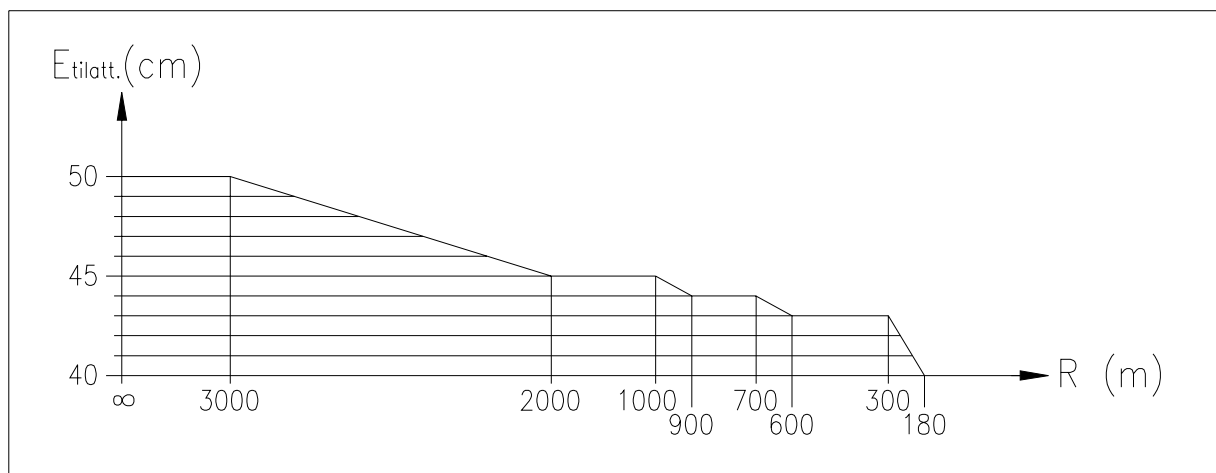
Figur 4 2 Vindutblåsningskurve for kontaktledningssystem med dimensjonerende hastighet over 200 km/h.
