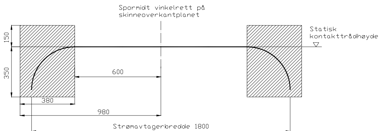
Figur 5.2 Klemmefritt rom (skravert), alle mål i mm.
