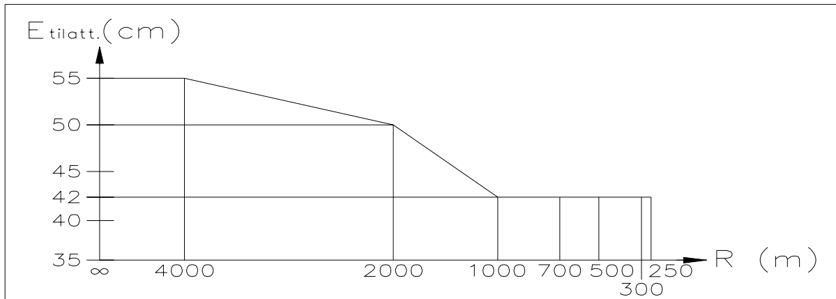
Figur 4 1 Vindutblåsningskurve for kontaktledningssystem med dimensjonerende hastighet opp til 200 km/h.
