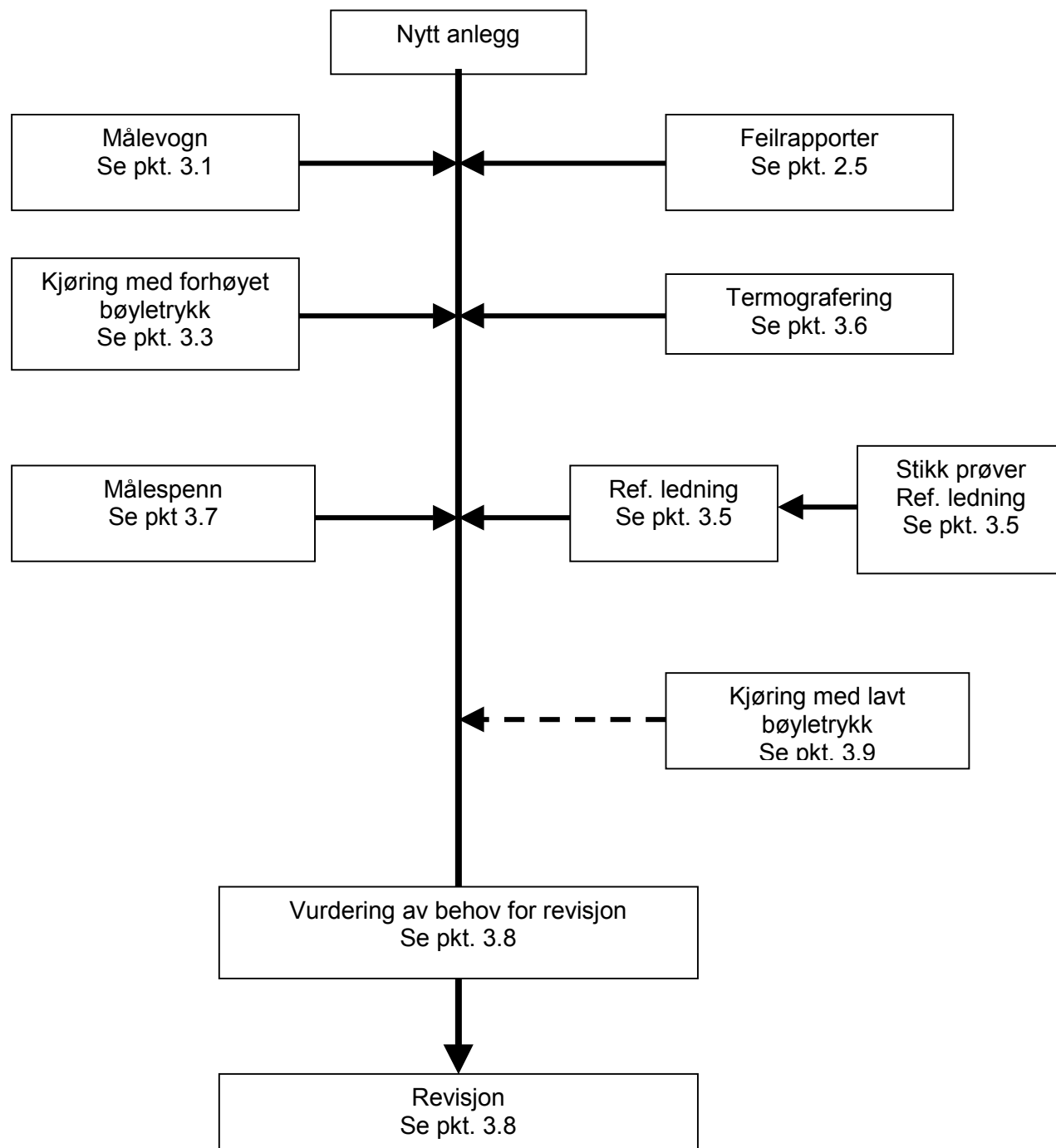
Figur 4.3 Flytskjema revisjoner
