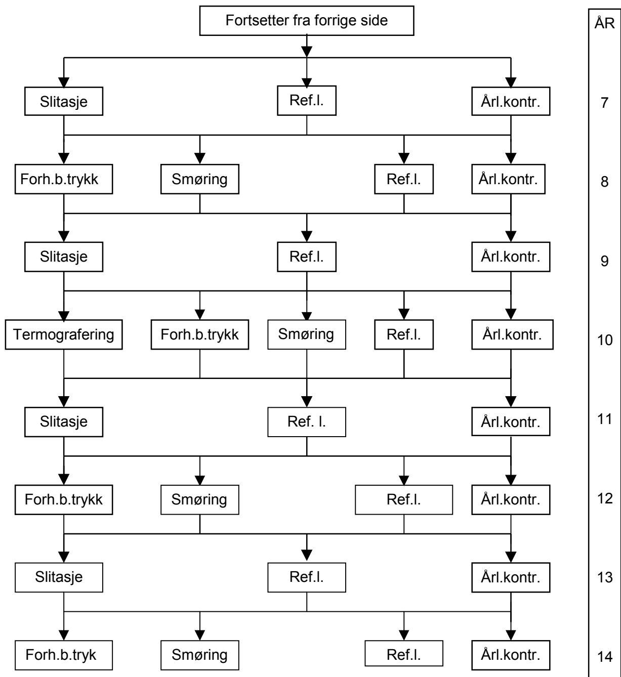
Fig. 4.2 Vedlikeholdsmatrise
