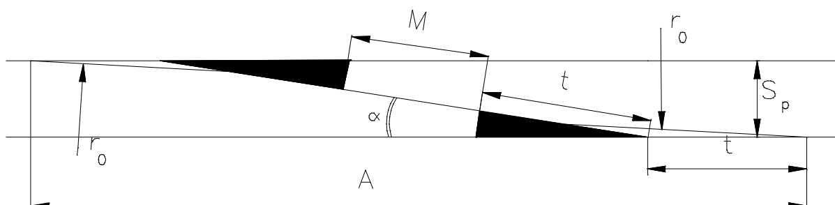
Figur 5.2 Sporsløyfe
