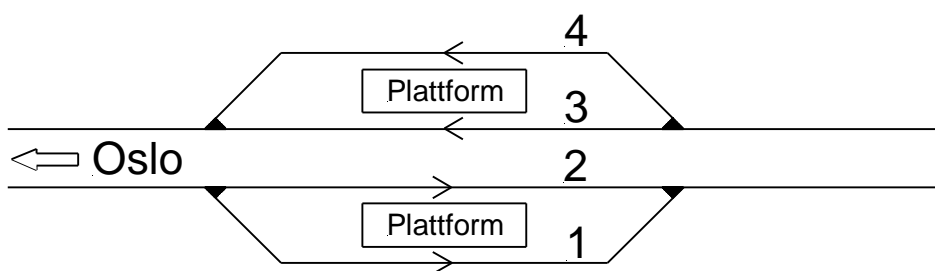
Figur 5.6 Eksempel på nummerering av stasjonsspor på dobbeltsporet strekning
