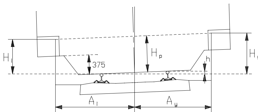
Figur 5.4 Spor med overhøyde
