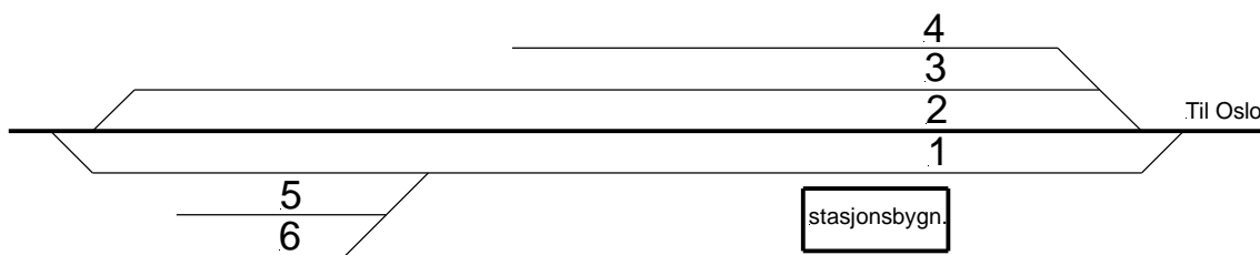
Figur 5.5 Eksempel på nummerering av stasjonsspor på enkeltsporet strekning
