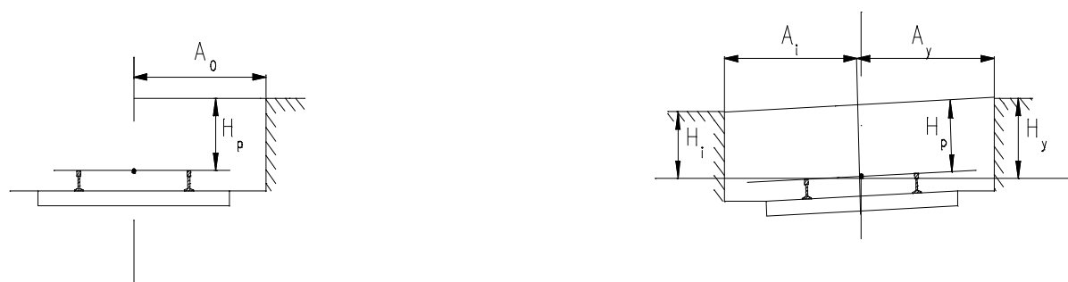
Figur 5.3 Plattformhøyder og avstand spormidt - plattformkant
