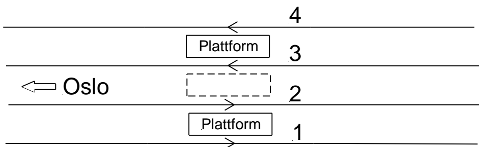
Figur 5.7 Eksempel på nummerering av stasjonsspor på strekning med 4 spor
