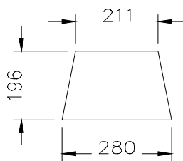
SNITT A-A
