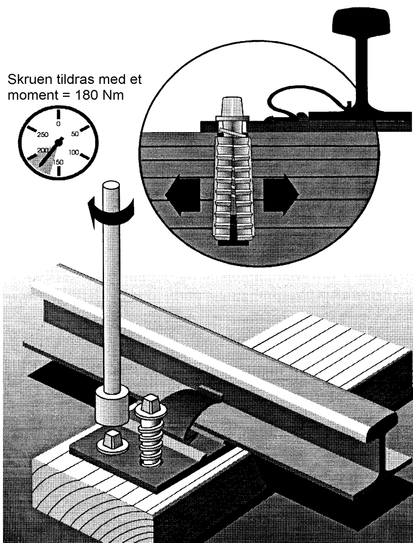
Nedskruing av svilleskrue
