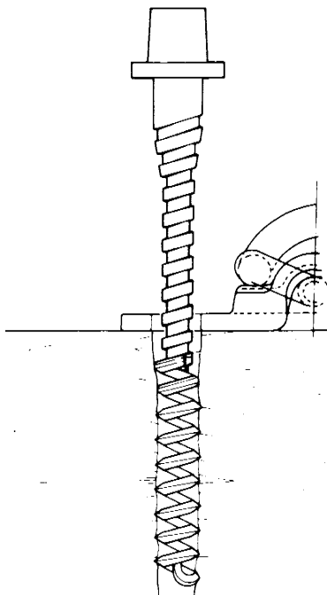
Figur 8.a.4 Fjerning av monteringsverktøy
