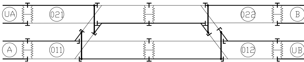
Figur 6.32 Stasjon på dobbeltsporet strekning, elektrifisert bane. Dobbeltisolert m/skinnebruksdeteksjon. Høyre/venstre hovedspor skal være elektrisk adskilt.
