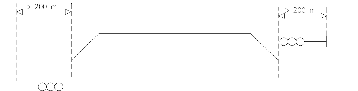
Figur 6.1 Plassering av innkjørhovedsignaler.
