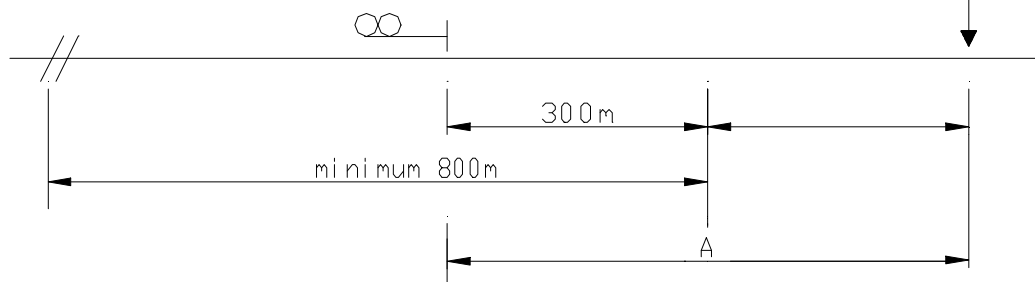
Figur 8.5 Veibomanlegg, plassering av innkoblingsfelter.
