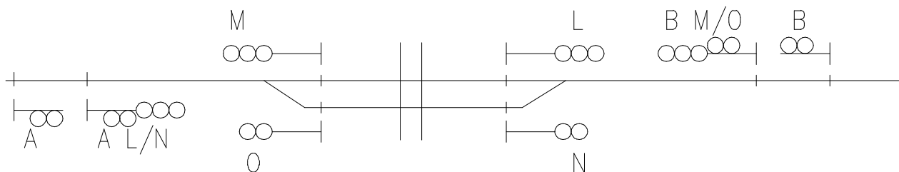
Figur 8.2 Planovergang mellom inn- og utkjørhovedsignalene.
