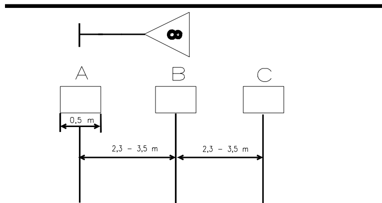
Figur 10.13 Baliseplassering ved hastighetssignaler.
