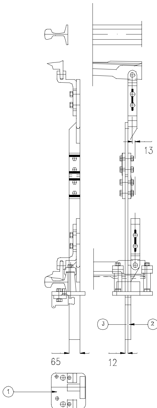
Skisse for sammenstilling av kontrollås.
