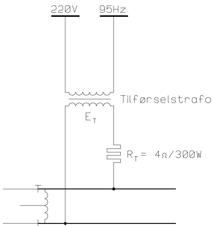
Figur 6.e.7 Tilførselkrets type 3.
