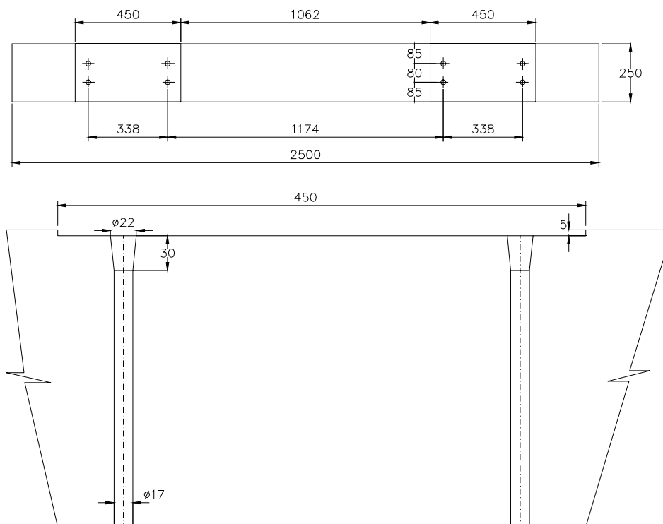
Figur 6.3 Bormønster for S49 med Pandrol befestigelse - Sk 3123
