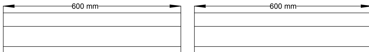
Figur 6.1 Prøveemner - skjøtsveising
