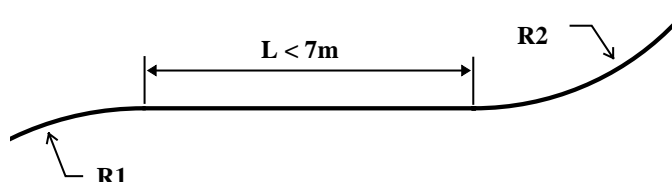
Figur 13.1 Overgangskurve med mellomliggende rettlinje < 7\text{m} .
