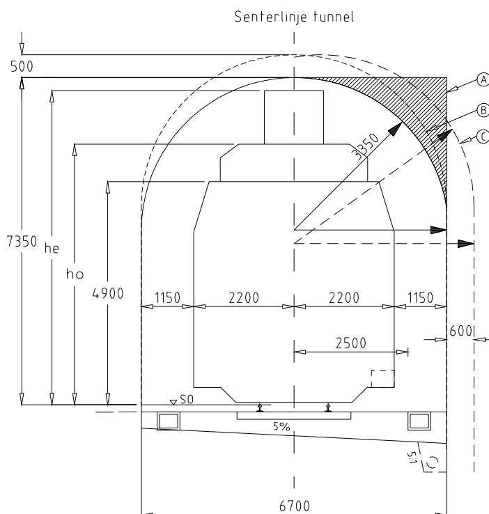
Normalprofil tunnel, enkeltspor
