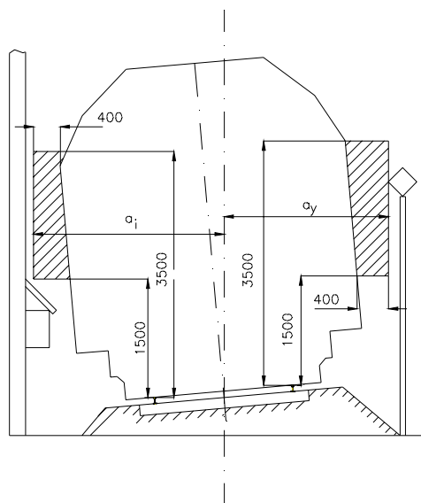
Figur 5.12 Avstand til master og andre gjenstander for A-85/96/C
