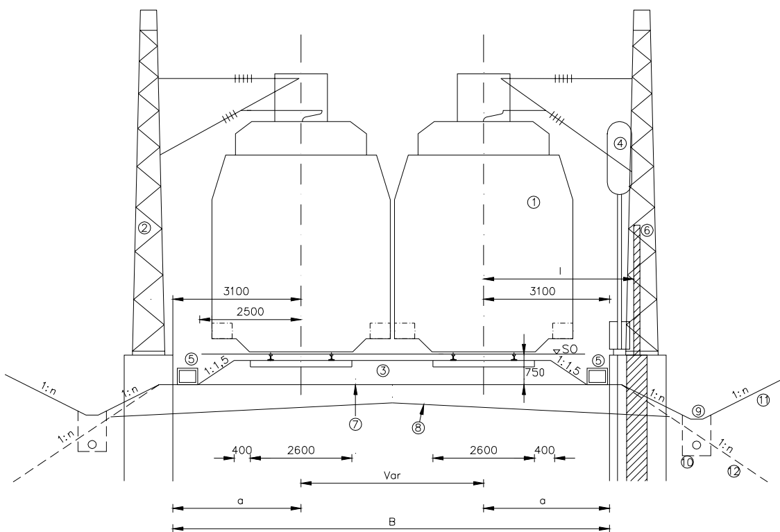
Figur 5.15 Normalprofil daglinje, dobbeltspor
